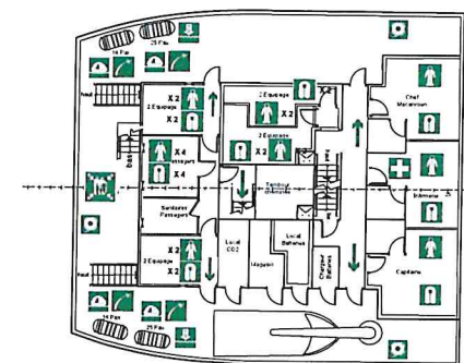
VUE 1 ER PONT
