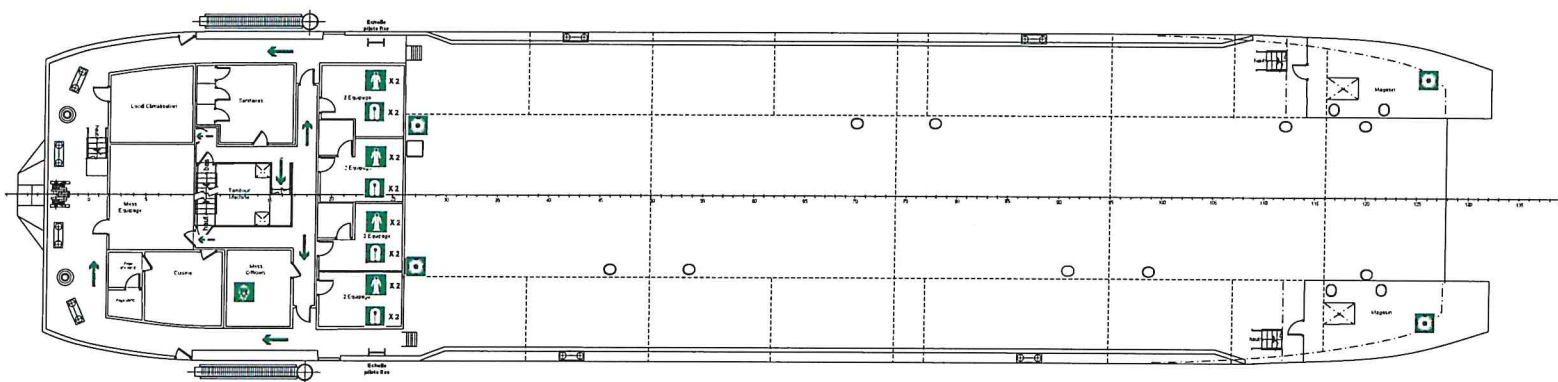
VUE PONT PRINCIPAL
